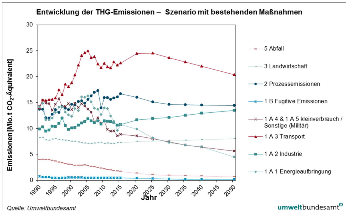
Abbildung 12: THG-Emissionen nach CRF-Sektoreinteilung (inkl. Emissionshandel)
