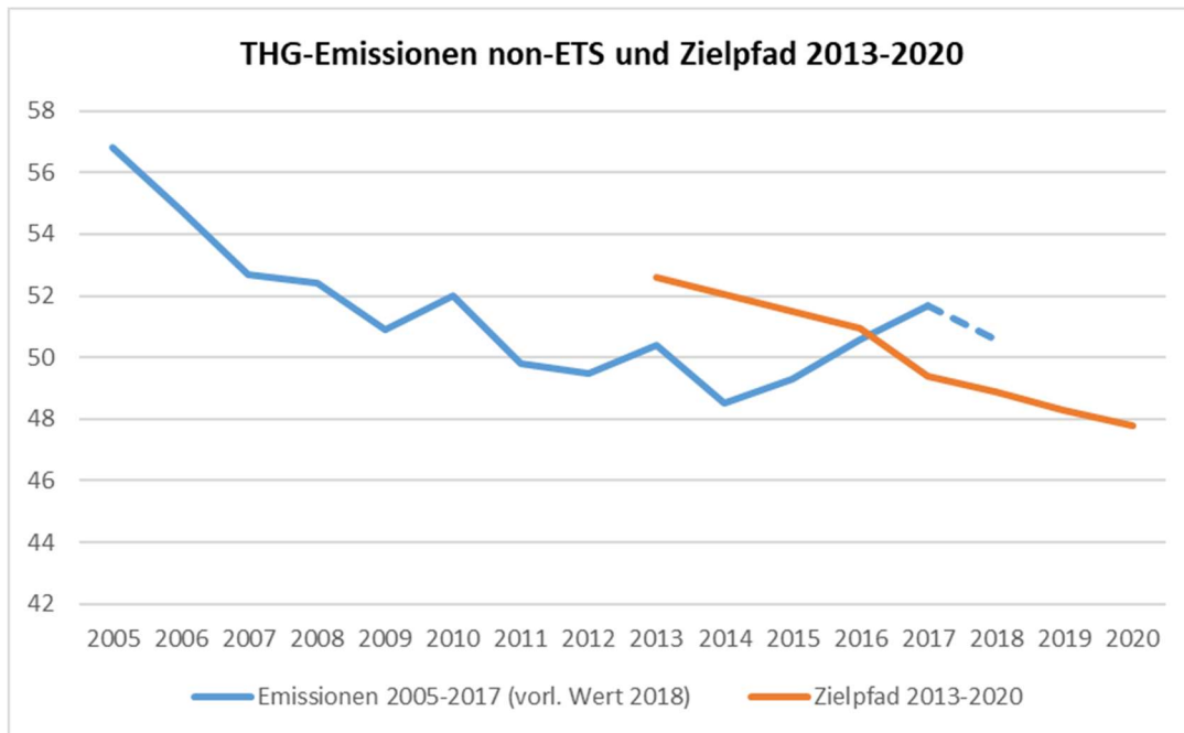
Abbildung 2: Treibhausgasemissionen Österreichs in Mio. t CO 2 -Äquivalent in Sektoren außerhalb des EU Emissionshandels 2005 bis 2017/2018 und Zielpfad 2013 bis 2020 nach Effort Sharing Entscheidung
