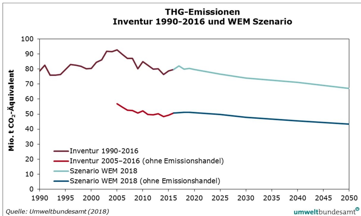
Abbildung 11: THG-Emissionen Inventur und WEM-Szenario mit und ohne EH
