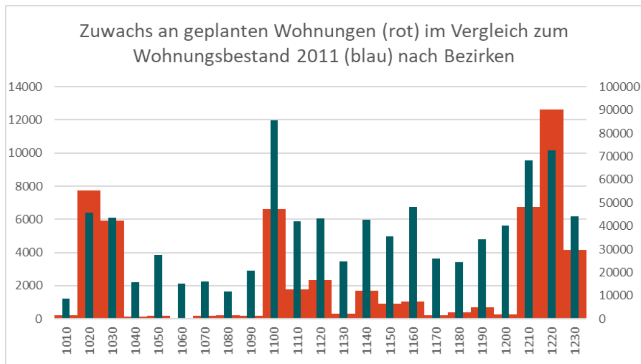
aller fertiggestellter und geplanter Wohnungen ab 2019 in EXPLOREAL (n = 54.689)
